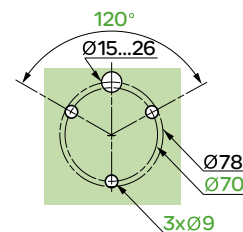
面板开孔
