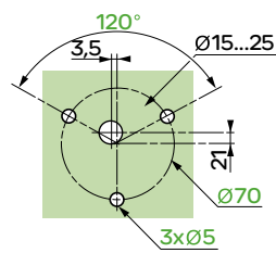
面板开孔
