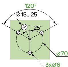
面板开孔
