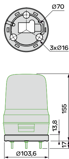
XVR Z082 (橡胶底座-可选件)
